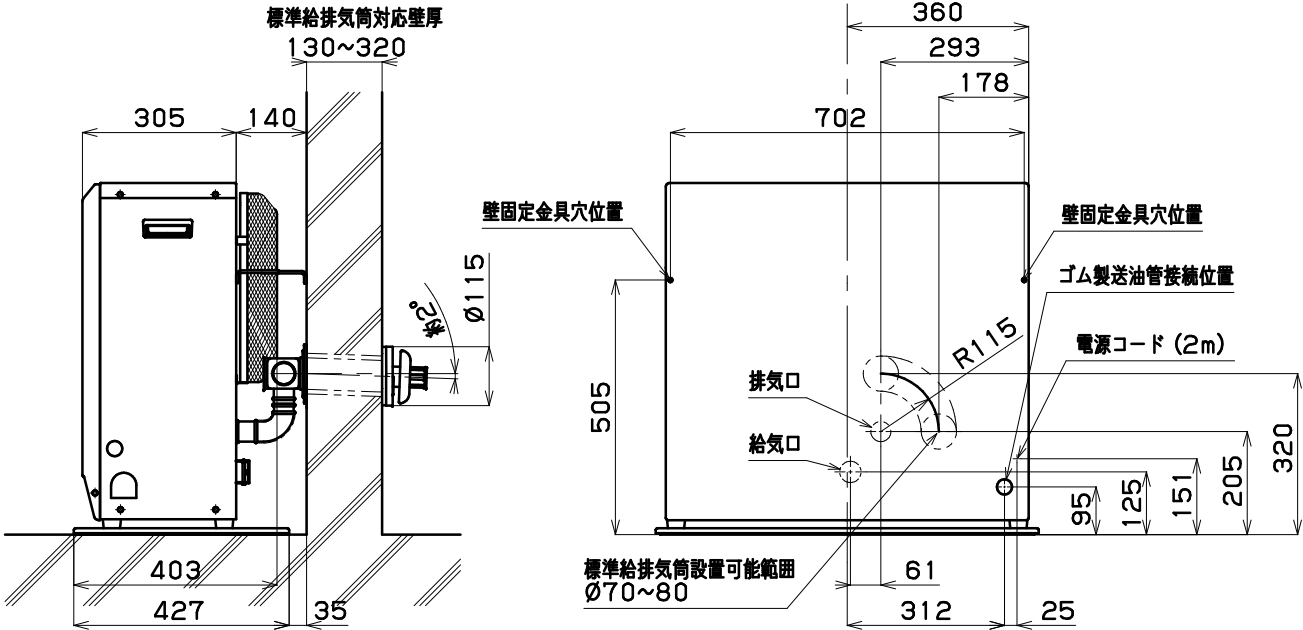
正面図
