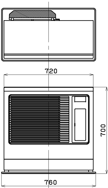
< 外形寸法図 >
