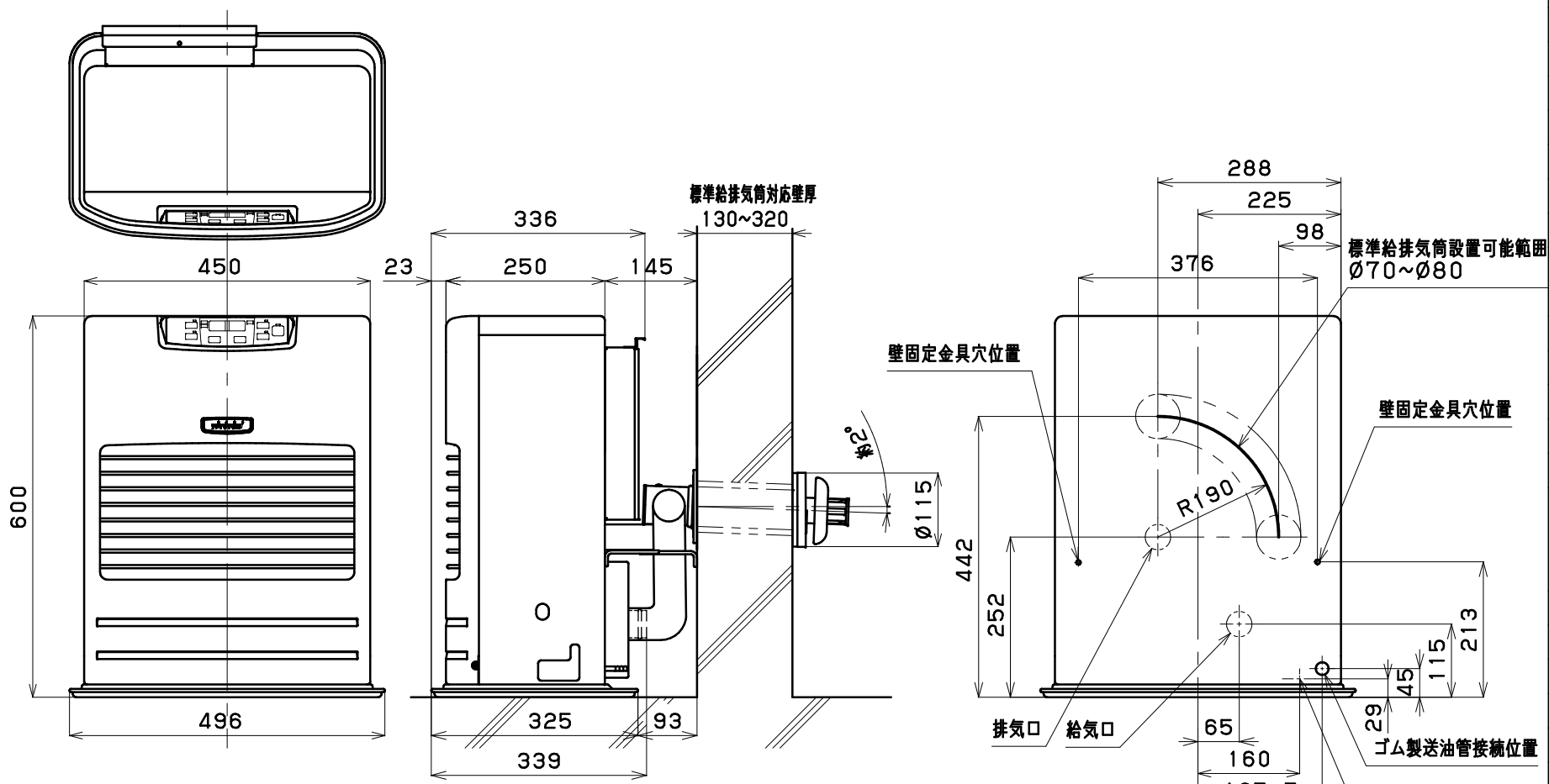
＜外形寸法図＞
