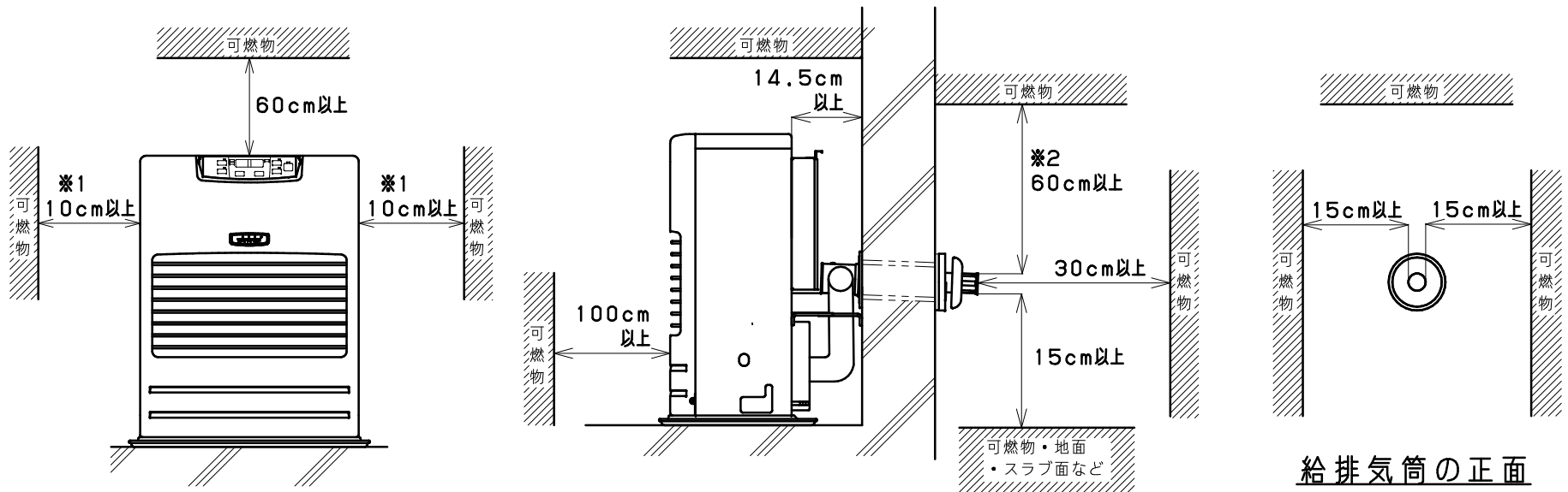
＜標準据付け例＞
