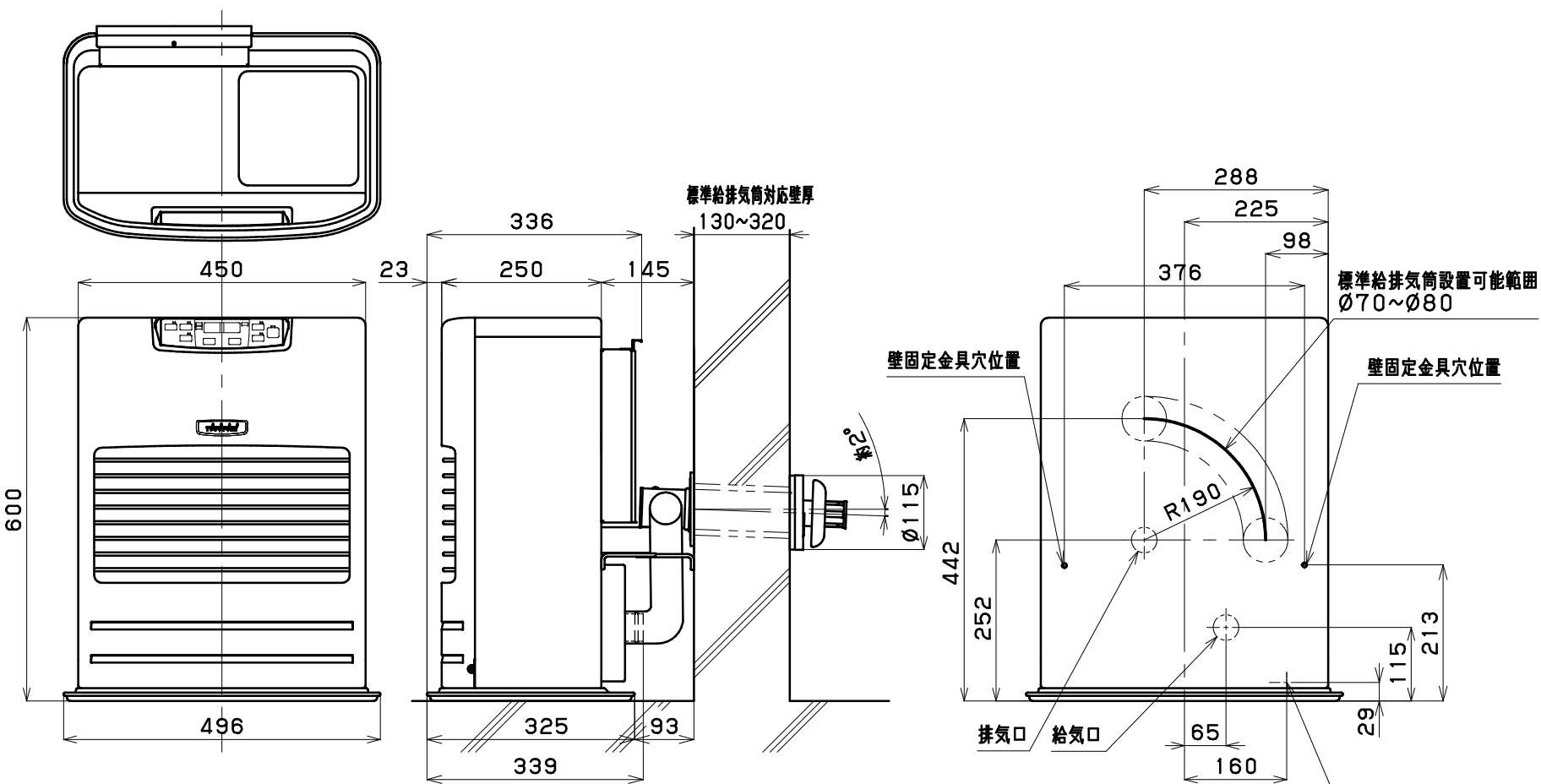
正面図
