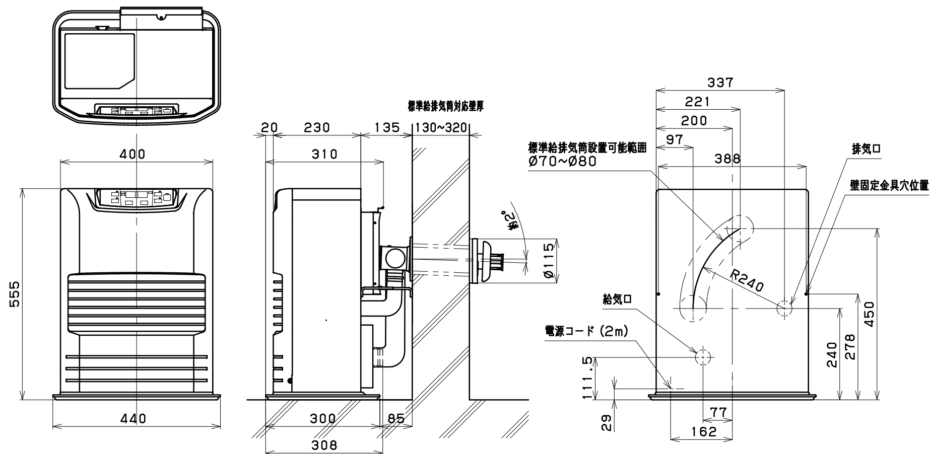
正面図
