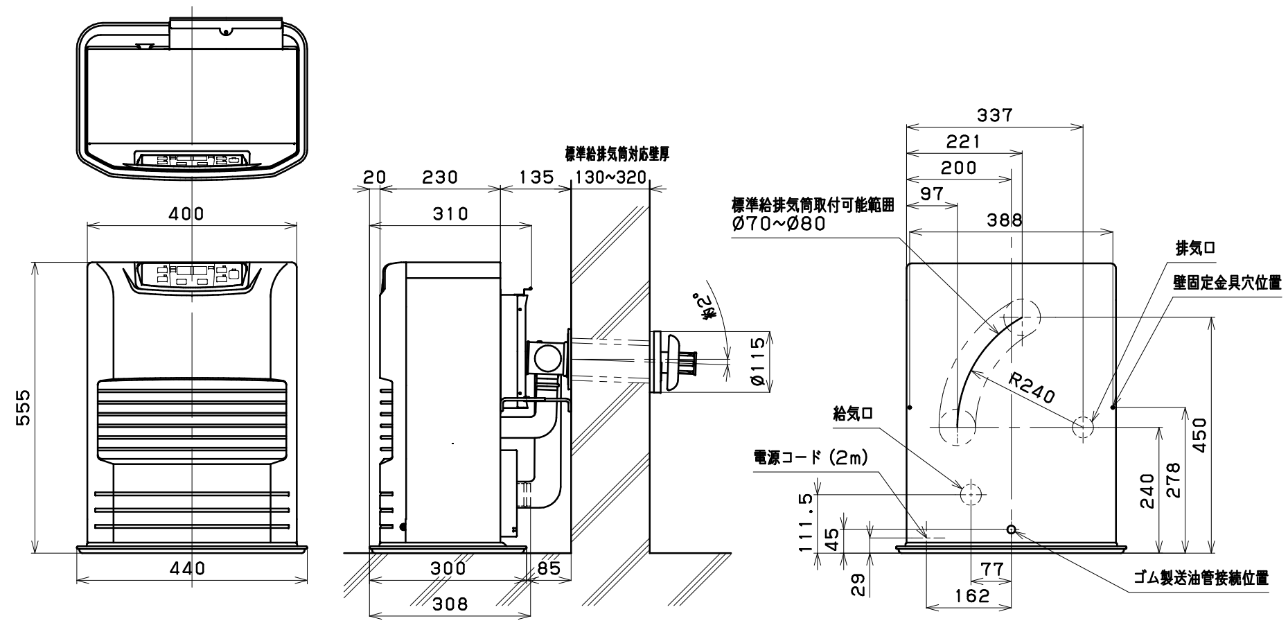
正面図
