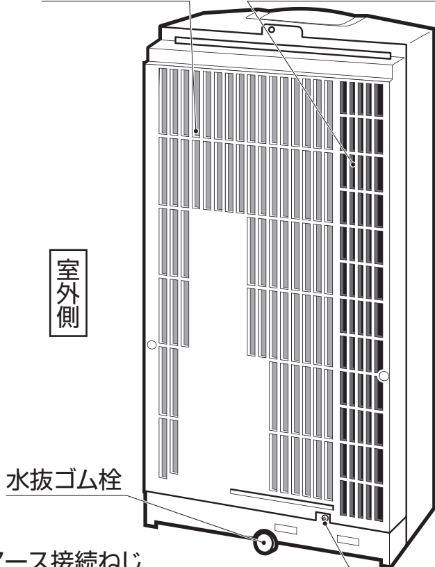
室外側吸込口 室外側吹出口(排熱)
