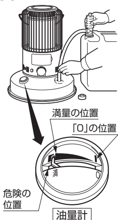
油量計
