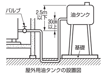
屋外用油タンクの設置図
