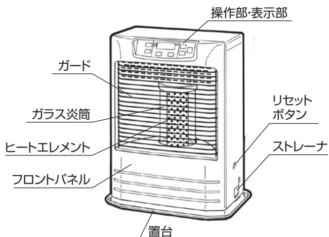
外観図
