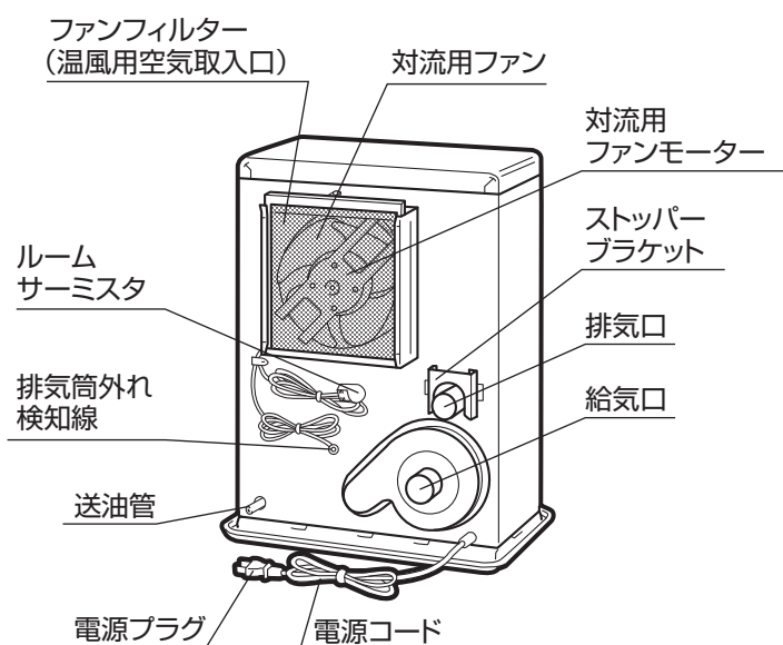
構造図
