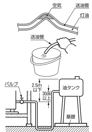
屋外用油タンクの設置図
