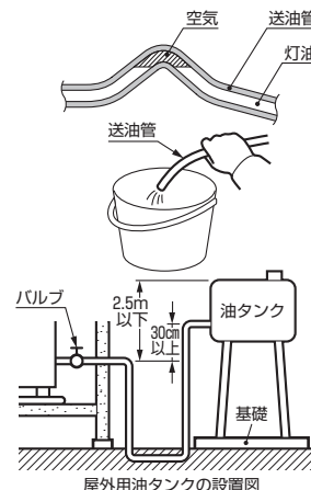
屋外用油タンクの設置図
