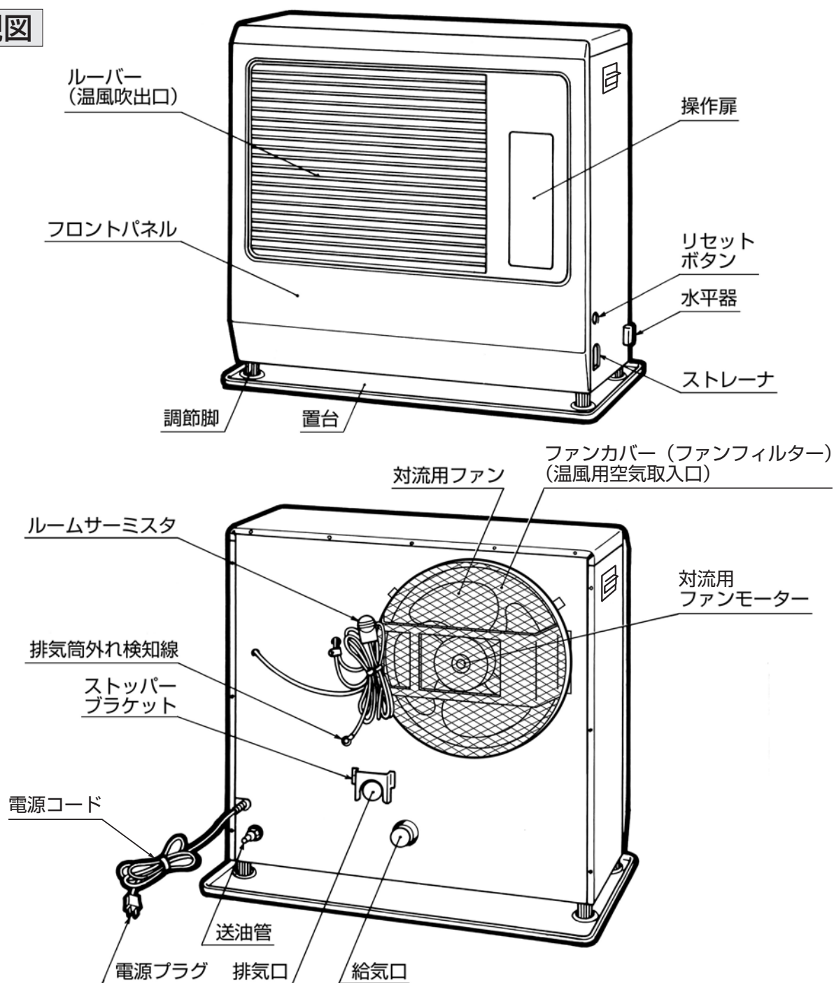
構造図
