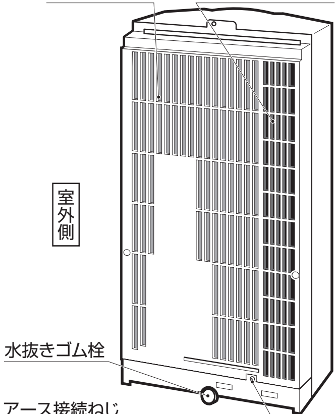
室外側吸込口 室外側吹出口(排熱)
