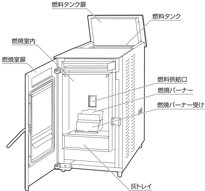
[内部構造図]
