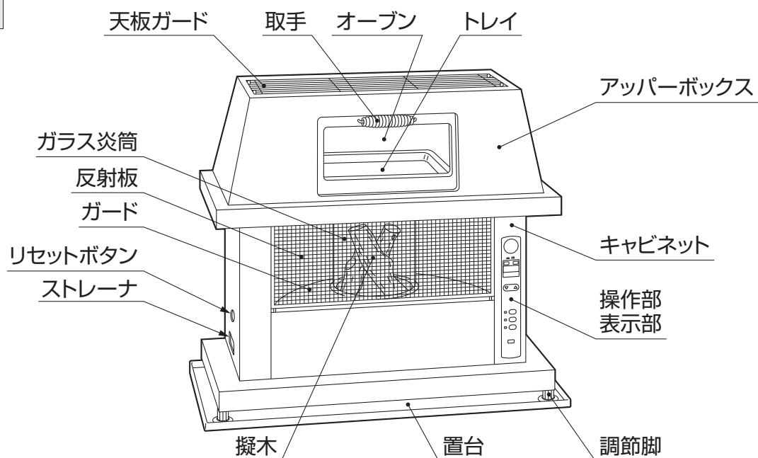
外観図
