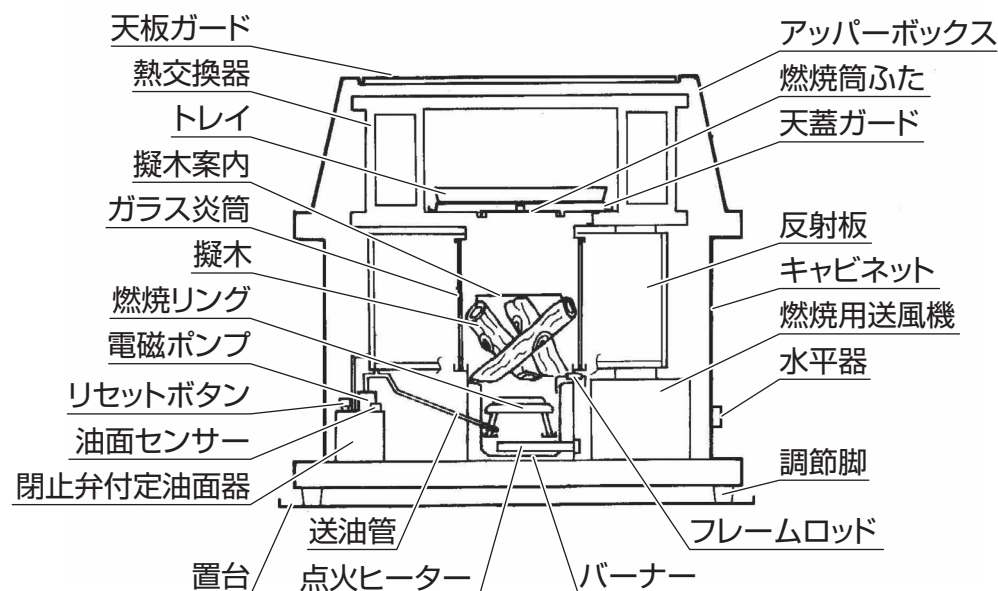
構造図
