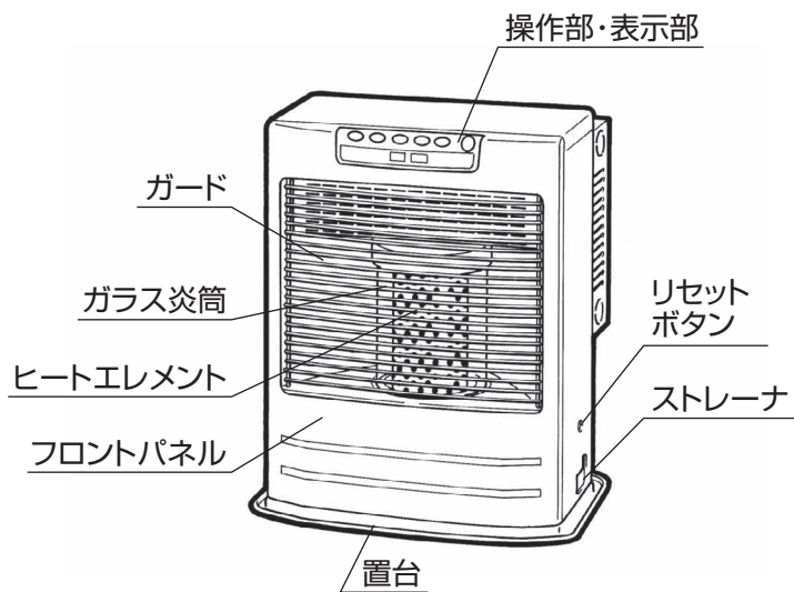
外観図 FR-S45B・FR-S55B
