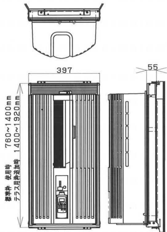
据付け枠取付状態
