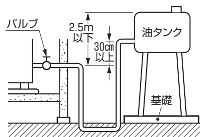
屋外用油タンク設置図
