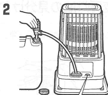
油量計
