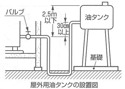
屋外用油タンクの設置図
