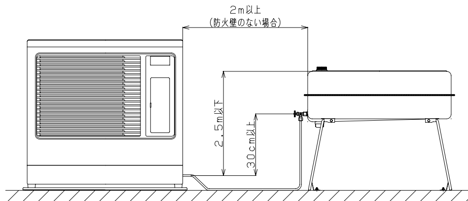
設置説明図
